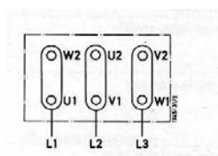
Fig.1.用于连接三相电机的 \Delta 接线图
